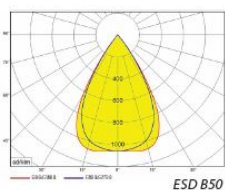
ESD B50
