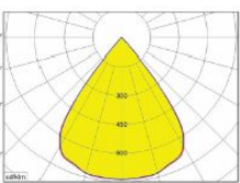
ESD B80
