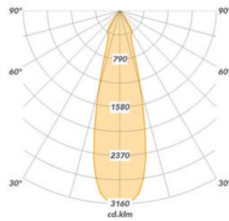
24° (2625-00011)
