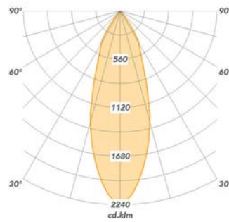
36° (2625-00012)
